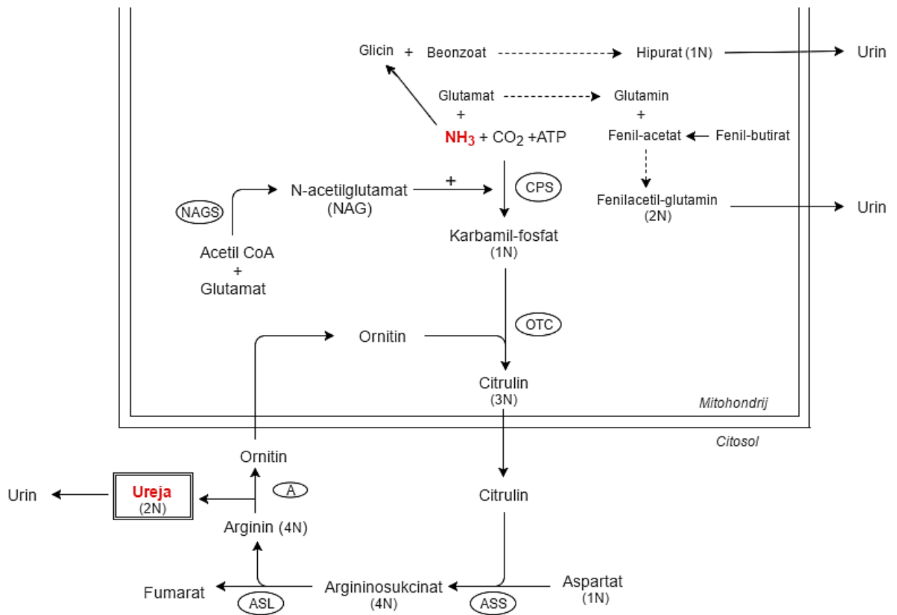
Slika 1. Ciklus sinteze ureje i alternativni metabolički putevi izlučivanja dušika. CPS-karbamil-fosfat sintetaza; OTC-ornitin transkarbamilaza; ASS-argininosukcinat sintetaza; ASL-argininosukcinat liaza; A-arginaza; NAGS-N-acetilglutamat sintetaza. Prema: Kliegman et al. (2015), str. 670.
