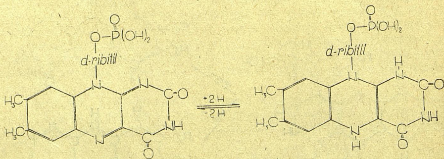
Dihidroizoaloksazin-mononukleotid
