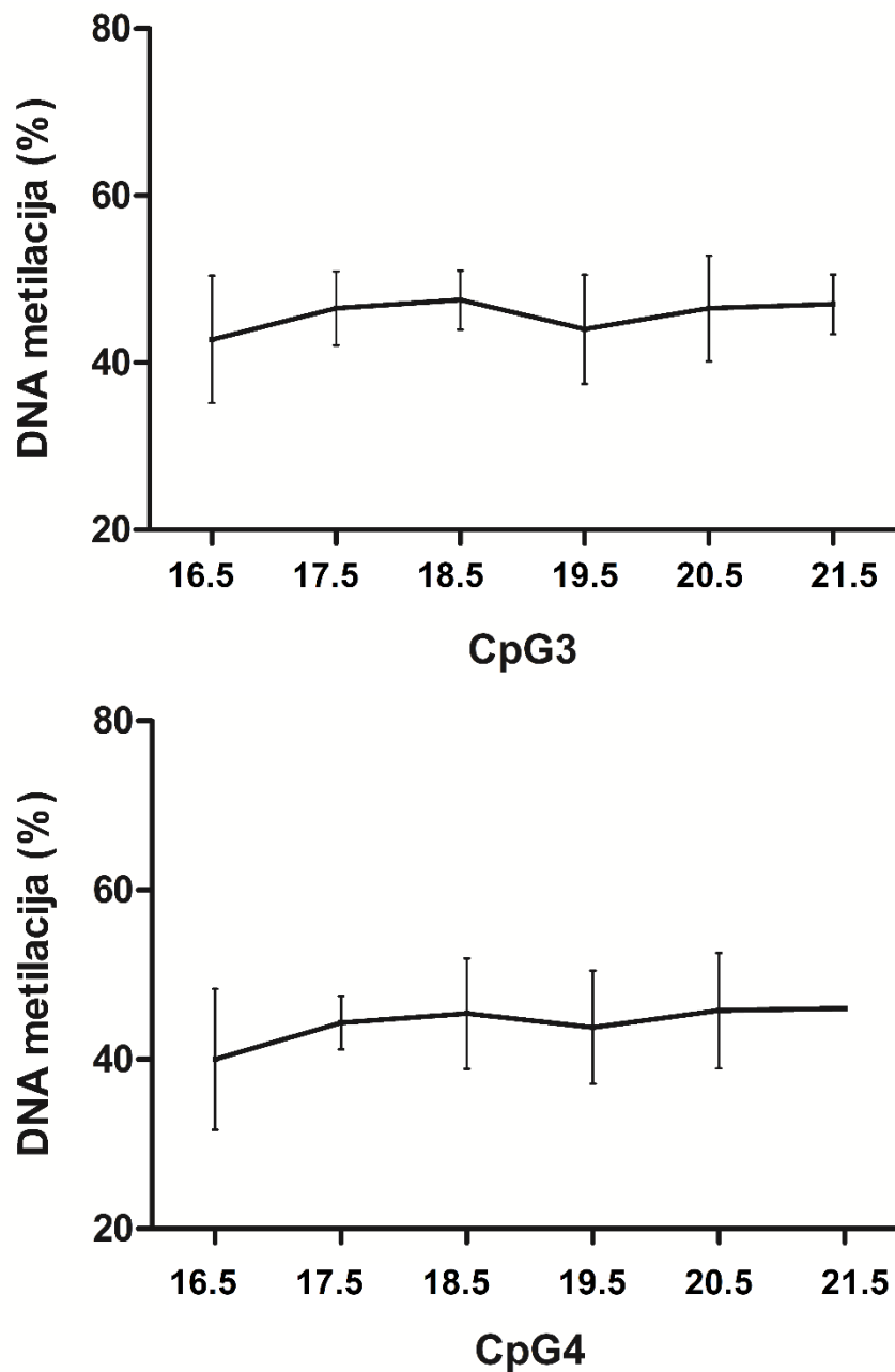
Slika 15. Postotak metilacije gena H19 na CpG3 (gore) i CpG4 (dolje) mjestu iz svježe smrznutih uzoraka štakorskih fetalnih sjemenika od 16.5 do 21.5 dpc. Kruskal-Wallis test s Dunnovim testom višestrukih usporedbi. Rezultati su prikazani kao srednja vrijednost \pm standardna devijacija. Broj uzoraka je minimalno 6 po skupini. Nema statistički značajne vrijednosti.
