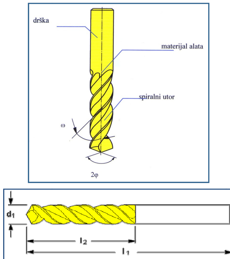
Slika 17. Spiralno svrdlo
