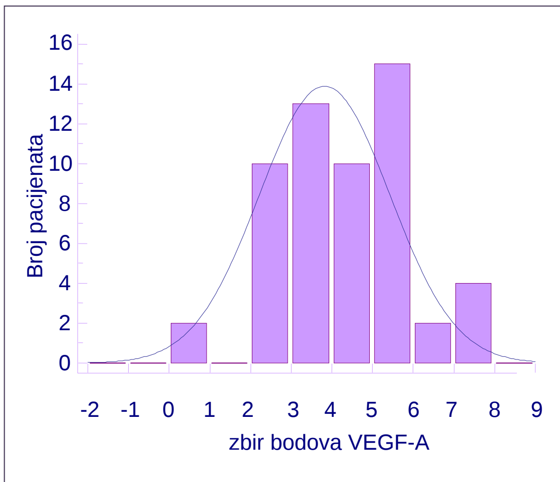
Slika 15. Histogram distribucije intenziteta imunoreaktivnosti (zbira bodova) VEGF-A. Kolmogorov-Smirnov test prihvata normalnost raspodjele ( P=0,185 )
