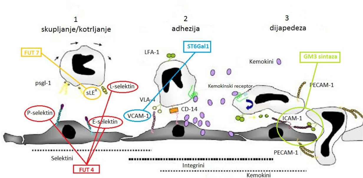
Slika 6.1. Shematski prikaz razvoja ateroskleroze i moguće uloge analiziranih glikoziltransferaza za koje su dobivene značajne razlike između skupina (preuzeto i modificirano od EAJ van Wanrooij, 2007.).
