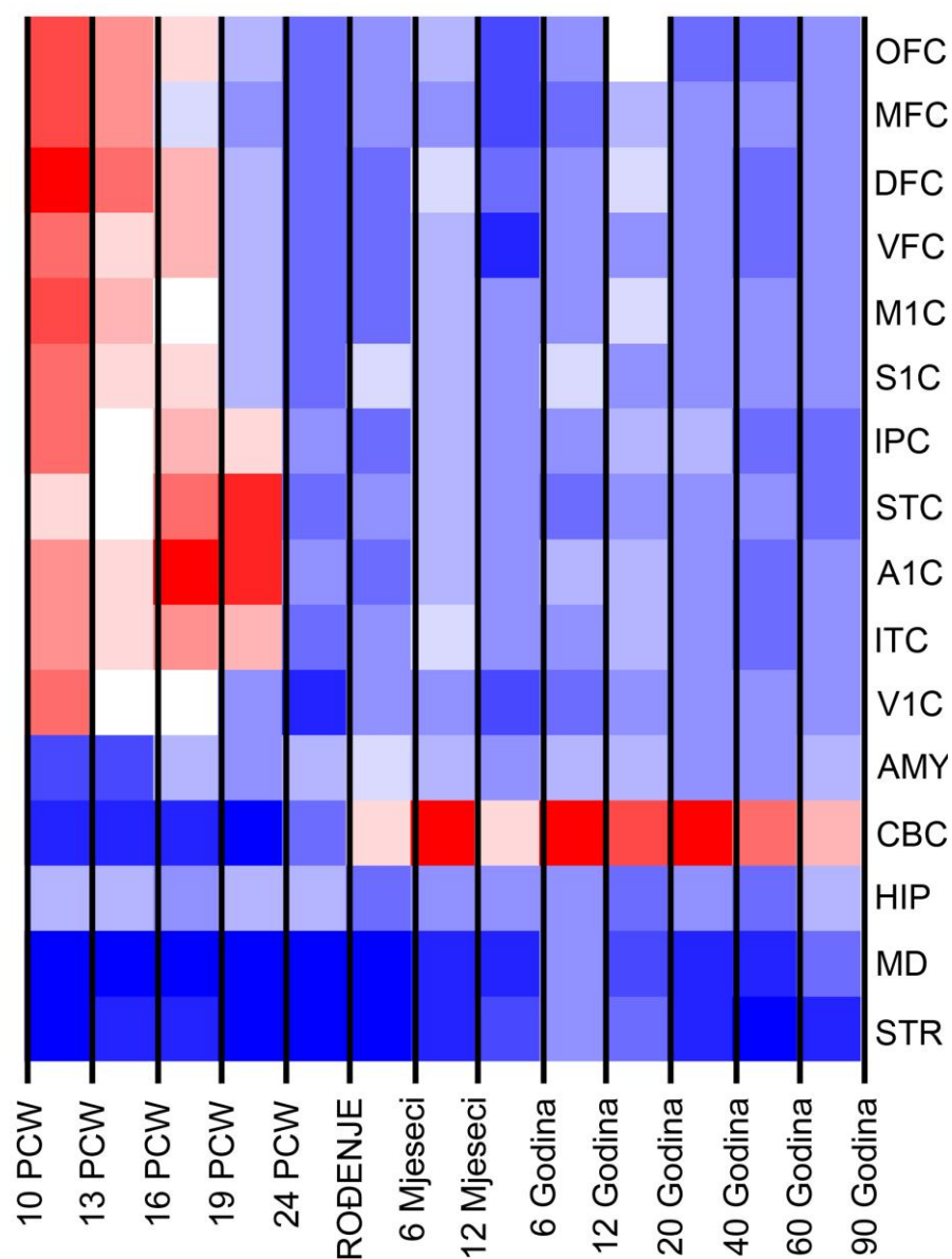
Slika 22. Ekspresija gena NURR1 u ljudskom mozgu. NURR1 nije eksprimiran u moždanoj kori nakon 19. postovulacijskog tjedna i tijekom cijelog života u AMY, HIP, MD, STR. U CBC postane eksprimiran nakon rođenja.
