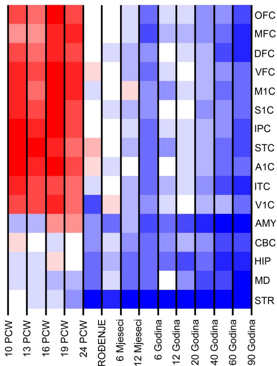
Slika 17. Ekspresija gena ADRA2A u ljudskom mozgu. ADRA2A je eksprimiran u visokim vrijednostima do 24. postovulacijskog tjedna, kada se počinje smanjivati na niže vrijednosti u odrasloj dobi.
