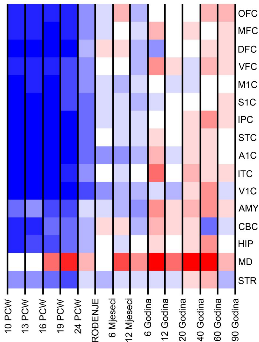
Slika 20. Ekspresija gena INPP4B u ljudskom mozgu. INPP4B nije eksprimiran u mozgu do 6. godine života, s iznimkom MD. Nakon 6. godine života, eksprimiran je u niskim vrijednostima.
