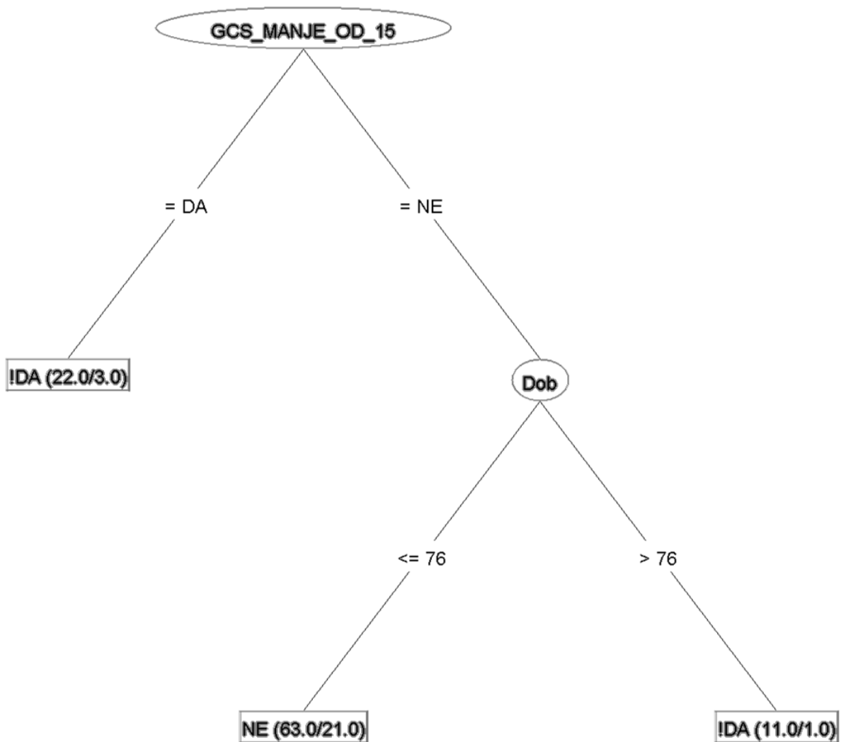
Slika 4. Stablo odlučivanja izvedeno J48 algoritmom u programu Weka, uz parametar generalizacije 10 [ ! DA - preminuli, NE - preživjeli, (x/y) : x - točno klasificirani bolesnici, y - netočno klasificirani bolesnici].
