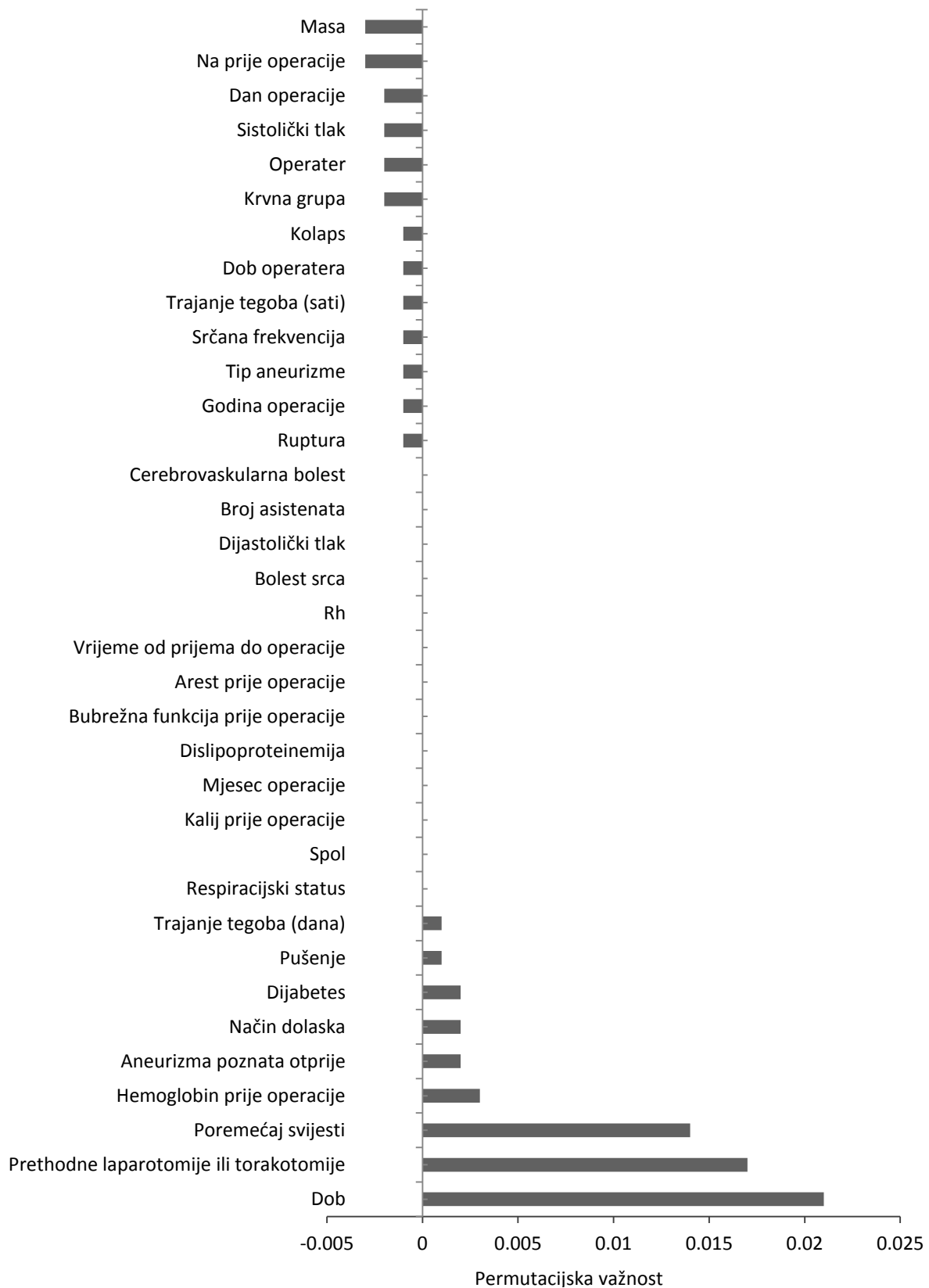
Slika 6. Permutacijska važnost varijabli u modelu slučajnih šuma.
