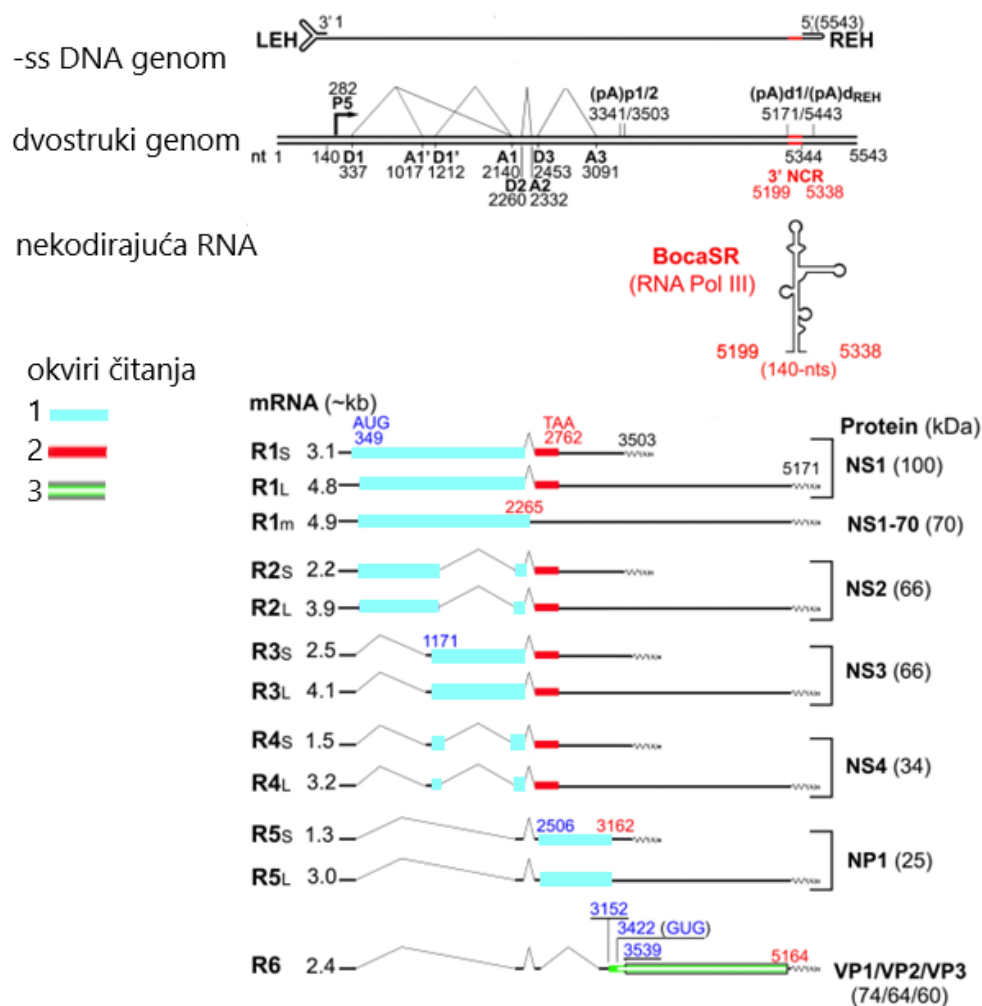
Slika 2. Transkripcijska karta HBoV 1. Prikazane su glavne transkripcijske oznake: ponavljajuće terminalne sekvence (LEH i REH), promotorska mjesta (P) te mjesta izrezivanja
