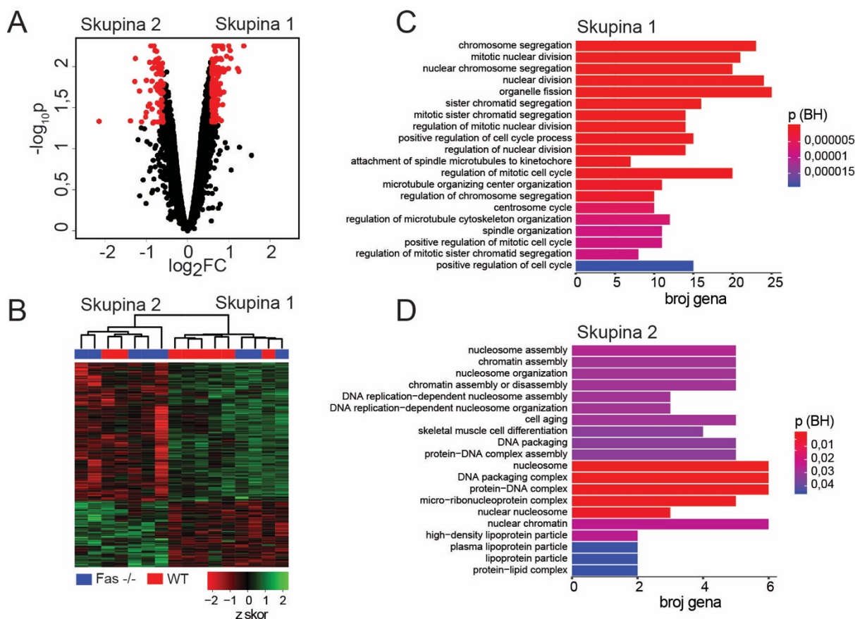
Slika 19. Analiza razlika u genskom izražaju skupina uzoraka razdvojenih na temelju hijerarhijske analize. Miševi su žrtvovani 10. dan nakon intra-artikularne injekcije metiliranog govedeg serumskog albumina (mBSA, prema engl. methylated bovine serum albumin ; AIA, prema engl. antigen induced arthritis ) ili fiziološke otopine puferirane fosfatom (PBS, prema engl. phosphate buffered saline ; CTRL). Nakon otpuštanja zglobnih stanica pomoću kolagenaze tipa IV, pomoću staničnog razvrstavanja aktiviranog fluorescencijom (FACS, prema engl. fluorescence-activated cell sorting ) izdvojena je populacija živih (DAPI - ) neeritroidnih (TER119 - ), nelimfoidnih (CD3B220NK1.1 - ) stanica, koje izražavaju biljege CD11b i Gr-1 (CD11b + Gr-1 low/+ ). Iz izdvojene mijeloidne populacije je potom izolirana ukupna stanična RNA, a po 4 pojedinačna uzorka zadovoljavajuće kvalitete iz svake pokuse skupine su fragmentirana, obilježena i hibridizirana na genske čipove GeneChip™ Mouse Gene 2,0 ST Array (Affymetrix). Nakon procijene kvalitete očitanih podataka bioinformatička analiza je provedena unutar sučelja Bioconductor u programu R. Analiza različito izraženih gena između dviju skupina uzoraka razdvojenih na temelju hijerarhijske analize provedena je pomoću algoritma limma (prema engl. linear models for microarray data ). U skupinu 1 svrstalo se 6 uzoraka miševa WT i 3 uzorka miševa Fas -/- , dok se u skupini 2 nalaze 5 uzoraka miševa Fas -/- i 2 uzorka miševa WT. (A) Rezultati su grafički prikazani odnosom negativnog logaritma prilagođene p vrijednosti ( -\log_{10}p ), i logaritma omjera promjene izražaja gena ( \log_2FC , prema engl. fold change), engl. volcano plot , pri čemu su pojedinačni geni prikazani crnim točkama, a crveno su označeni geni zadovoljavajuće prilagođene p vrijednosti ( p < 0,05 , Benjamini-Hochberg) te omjera promjene (apsolutni FC > 1,5 ). (B) Razlike u izražaju također su prikazane toplinskom mapom (prema engl. heatmap ) u kojoj su zelena boja predstavlja višu a crvena nižu razinu izražaja gena. Pomoću analize zastupljenosti GO termina određene su biološke funkcije, stanične komponente i molekularni procesi pojačano zastupljeni među genima pojačano izraženima u (C) skupini 1 i (D) skupini 2. Stupci za svaki od 20 najznačajnije promijenjenih GO termina prikazuju broj gena koji pripadaju pojedinom GO terminu, a boja stupca odgovara prilagođenoj p vrijednosti ( p < 0,05 , Benjamini-Hochberg).
