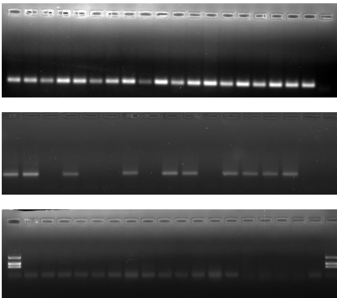
Slika 10. Gelovi agaroze s beta aktin (vrh), SPF+T7/SP6 (sredina) i amplikonima specifičnim za HPV tipove 16, 18 i 33 u kombiniranoj reakciji (dolje).
