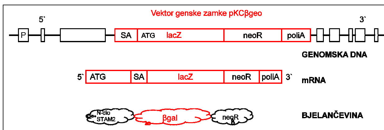
Slika 4. Shematski prikaz ugradnje vektora genske zamke pKC199βgeo u intron između 2. i 3. egzona gena Stam2 . Pomoću primača prekrajanja (SA, engl. splice acceptor ) i start kodona (ATG - inicijator transkripcije) vektor ostaje ugrađen u mRNA. Budući da vektor na svom 3' kraju posjeduje poliadenilacijski signal (poliA) dolazi do prekida transkripcije nizvodno od signala. Ukoliko je promotor (P) gena Stam2 aktivan, dolazi do stvaranja stopljene bjelančevine sastavljene od 14% N-kraja bjelančevine STAM2, β-galaktozidaze (β-gal) i neomicin fosfotransferaze (neoR).
