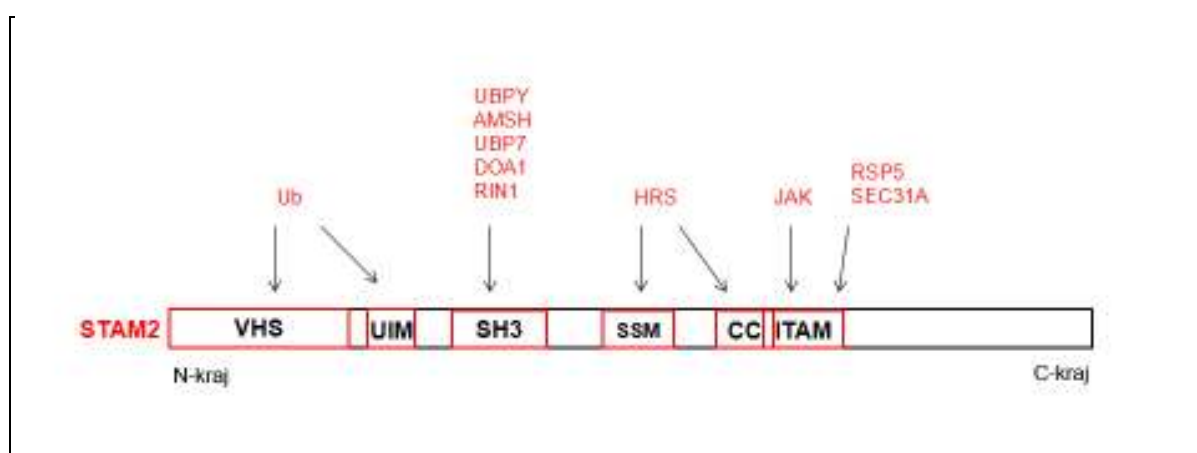
Slika 1. Shematski prikaz građe bjelančevine STAM2 s domenama VHS, UIM, SH3, SSM, CC i ITAM, te bjelančevina koje se vezuju za pojedine domene STAM2.
