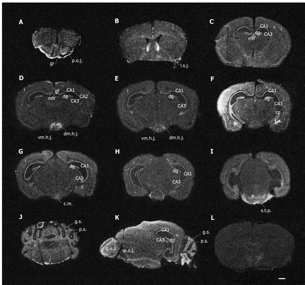
Slika 10. Izražaj gena Stam2 u mozgu odraslog miša. (A - K) Serijski koronarni kriorezovi odraslog mozga miša divljeg tipa koji posjeduje normalan gen Stam2 . (L) Koronarni kriorez mozga miša divljeg tipa tretiran „sense“ sandom, koja predstavlja negativnu kontrolu. p.o.j. - prednja olfaktorna jezgra, gr - granularni sloj olfaktornog bulbosa, g.o.b. - glavni olfaktorni bulbus, l.s.j. - lateralne septalne jezgre, vm.h.j. - ventromedijalna hipotalamička jezgra, dm.h.j. - dorzomedijalna hipotalamička jezgra, mh - medijalna habenula, i - izokorteks, CA1,CA2,CA3 - cornu ammonis , dg - dentatni girus, gf - gyrus fasciolaris , s - subikulum, j.a. - jezgre amigdale, cp - caudoputamen, cm - corpus mamillare , p - pons, s.t.p. - siva tvar ponsa, p.s. - sloj Purkinjeovih stanica, g.s. - granularni sloj malog mozga. Crta mjerila - 1 mm.
