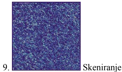
Slika 1. Pregled metode analize genskih mikročipova
