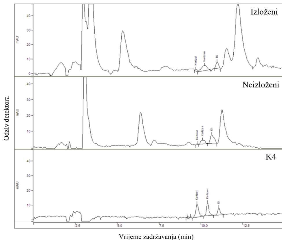
Slika 4.12. Kromatogrami koncentriranih ekstrakata poduzoraka slina izloženih i kontrolnih sudionika te kalibracijske otopine K4
