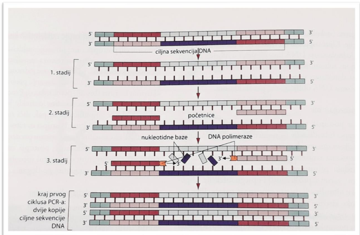
Slika 2. Lančana reakcija polimerazom za amplifikaciju specifične sekvencije DNA (preuzeto iz: Kalenić S i sur. Medicinska mikrobiologija. Zagreb: Medicinska naklada; 2013.)
