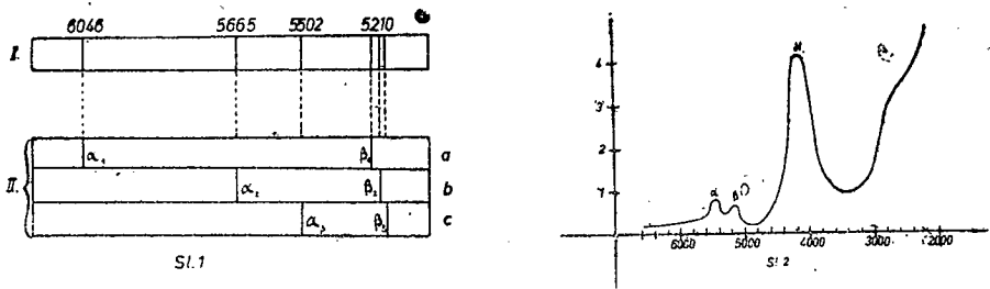
Sl. 1. — I. Spektar potpunog reduciranog citokroma iz kvasca, II. Disocijacija tog spektra na njegova tri sastavna dijela: citokrome a, b, c.
