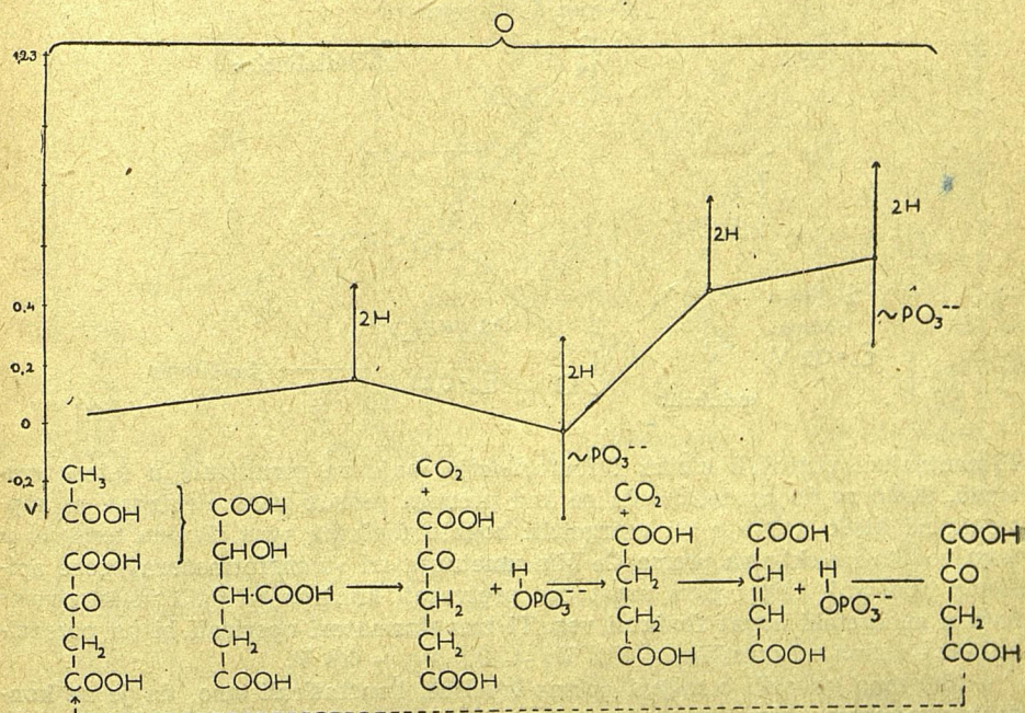
Shema 4. (Lipmann)
