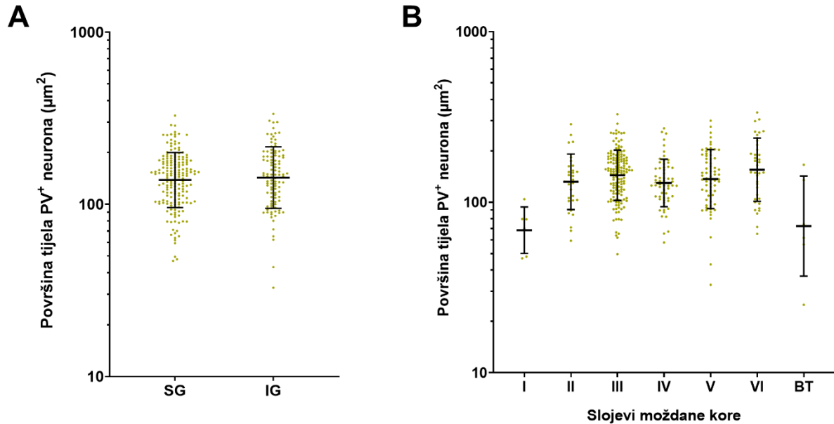
Slika 5.30. Točkasti dijagrami raspršenja s prikazom raspodjele površine tijela PV + neurona na logaritamskoj skali (zbirni podatci za Brodmannova polja 9 i 14r). Dugačke horizontalne crte predstavljaju geometrijsku sredinu, a stupci pogreške GSD. (A) Usporedba površine tijela PV + neurona između supragranularnih i infragranularnih slojeva. (B) Raspodjela površine tijela PV + neurona po slojevima moždane kore.
