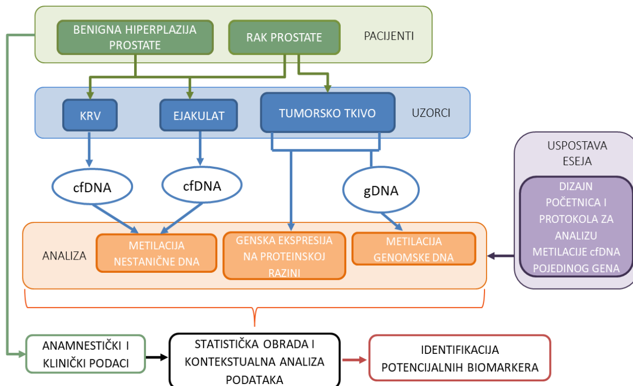
Slika 10. Dizajn istraživanja.
