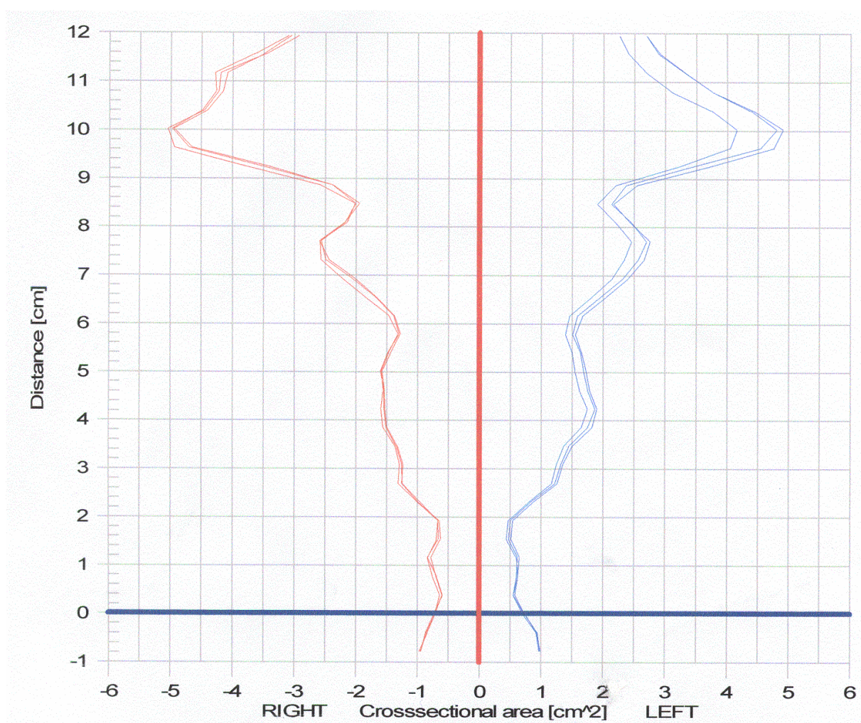
Slika 17. Prikaz AR krivulje u obliku linearne skale, pri čemu je na y-osi prikazana aksijalna udaljenost od nosnica do koana izražena u cm, a na x-osi površina poprečnog presjeka nosne šupljine izražena u \text{cm}^2
