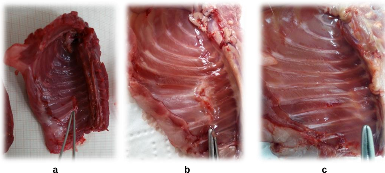
Slika 17. Makroskopski nalaz na mjestu učinjenih fraktura rebra 20-ti dan nakon frakture rebra (a – manja ožiljna reakcija na mjestu fraktura kod kontrolne skupine, b – izraziti ožiljak kod životinja tretiranih s L-NAME, c – gotovo bez ožiljka kod životinja tretiranih s BPC 157).
