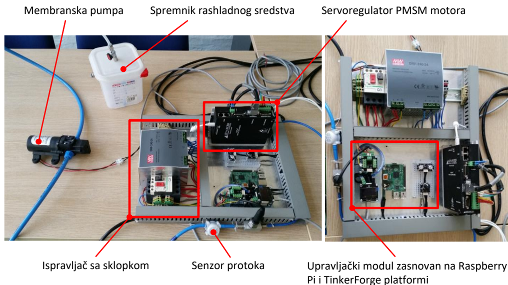
Slika 29. Sustav za regulaciju protoka rashladnog sredstva (PMSM – permanent magnet servo motor)
