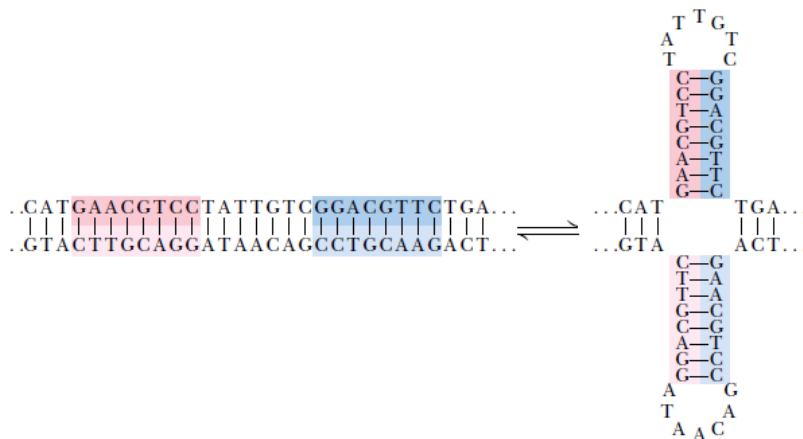
Slika 7.2-4 Formiranje križne strukture iz palindromske sekvence unutar DNA. Samokomplementarna obrnuta ponavljanja se mogu rearanžirati za dobivanje vodikovim vezama povezane križnih struktura. (Garrett & Grisham, 2012, str. 378)
