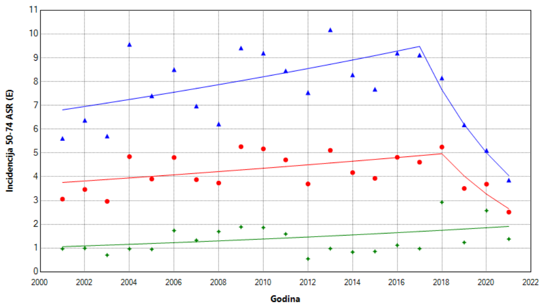
Slika 7 Joinpoint analiza incidencije mezotelioma za osobe u dobi od 50 do 74 godina u Republici Hrvatskoj u razdoblju od 2001. do 2021. godine (ASR (E) - dobno standardizirane stope - korišteno Standardno europsko stanovništvo; trokut - muškarci; krug - ukupno; romb - žene).
